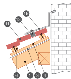
Примыкание кровли к стене
