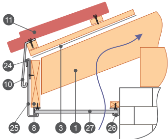
Подшивка свеса
